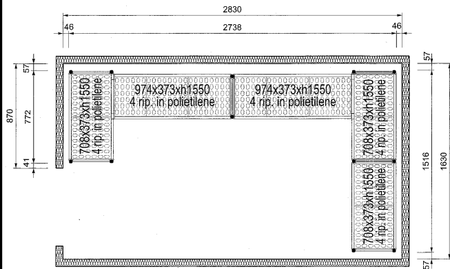
Boven aanzicht
